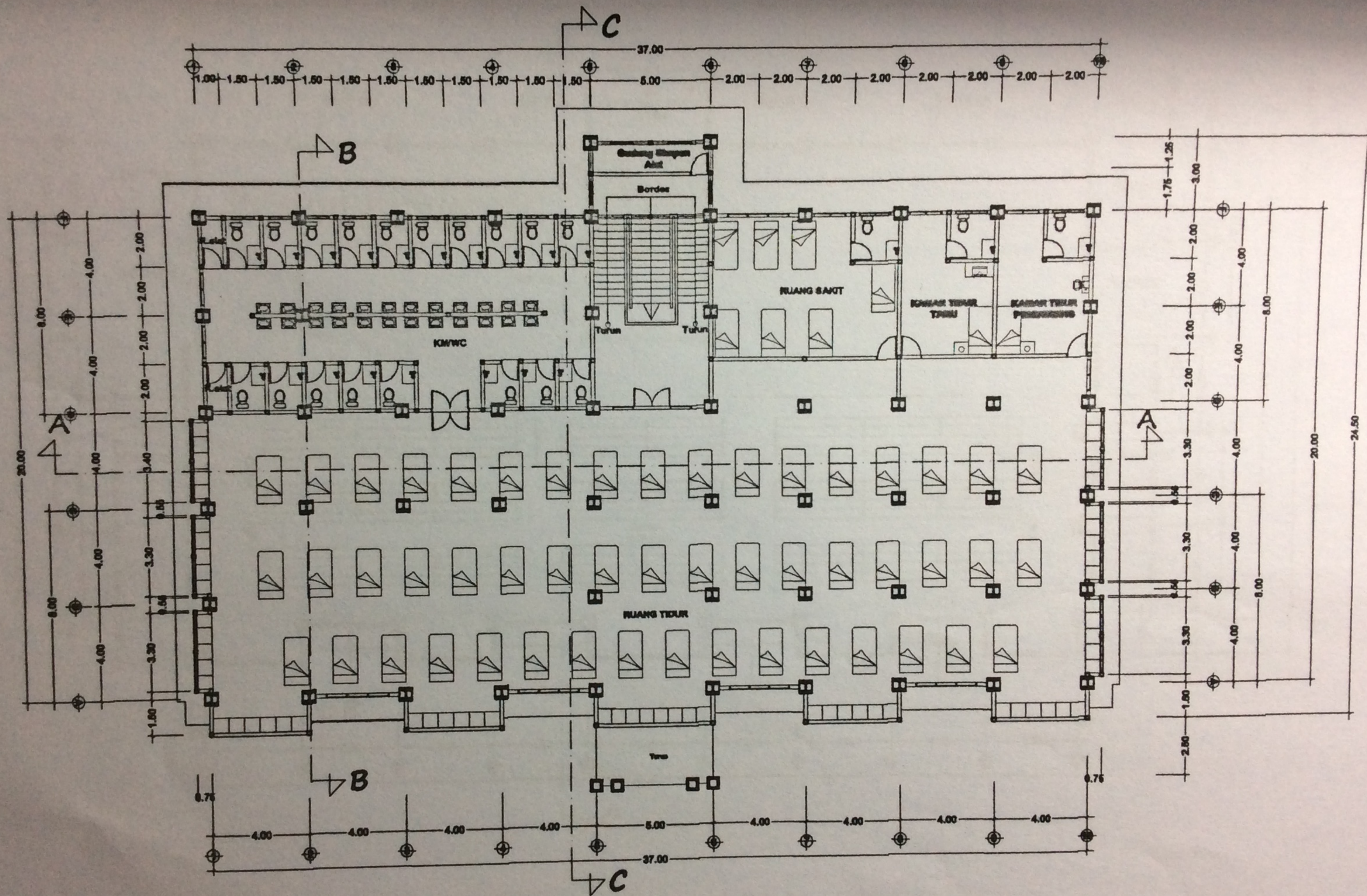
R DENAH LT. II Skala 1 : 200
