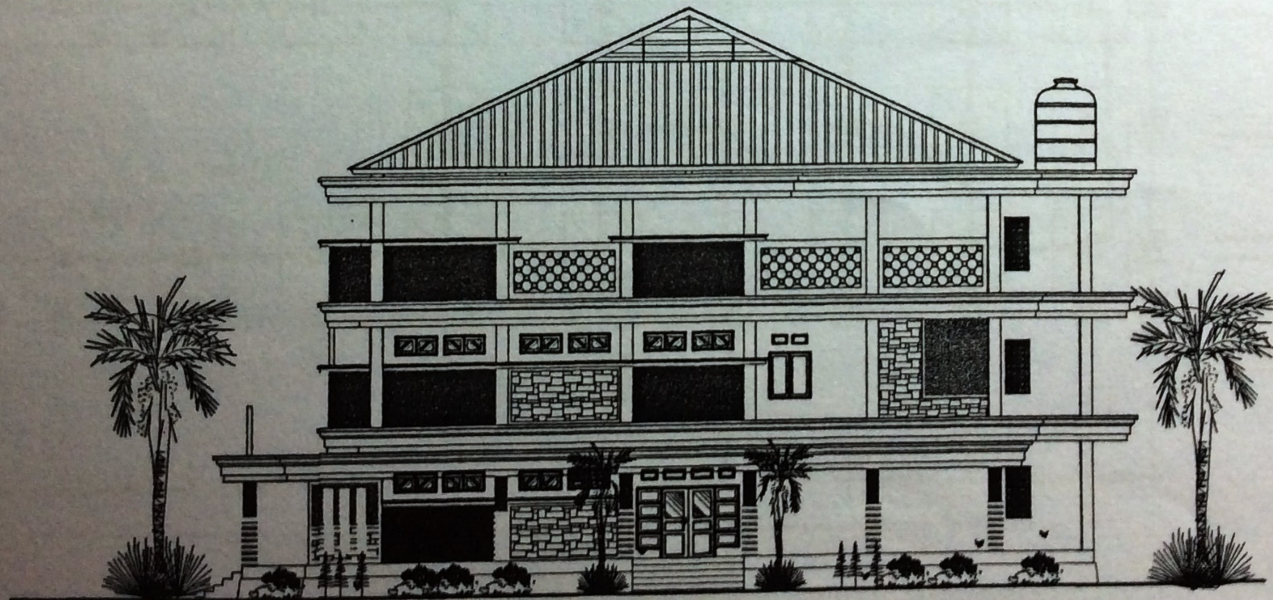
TAMPAK SAMPIK KANAN Skala 1 : 200
