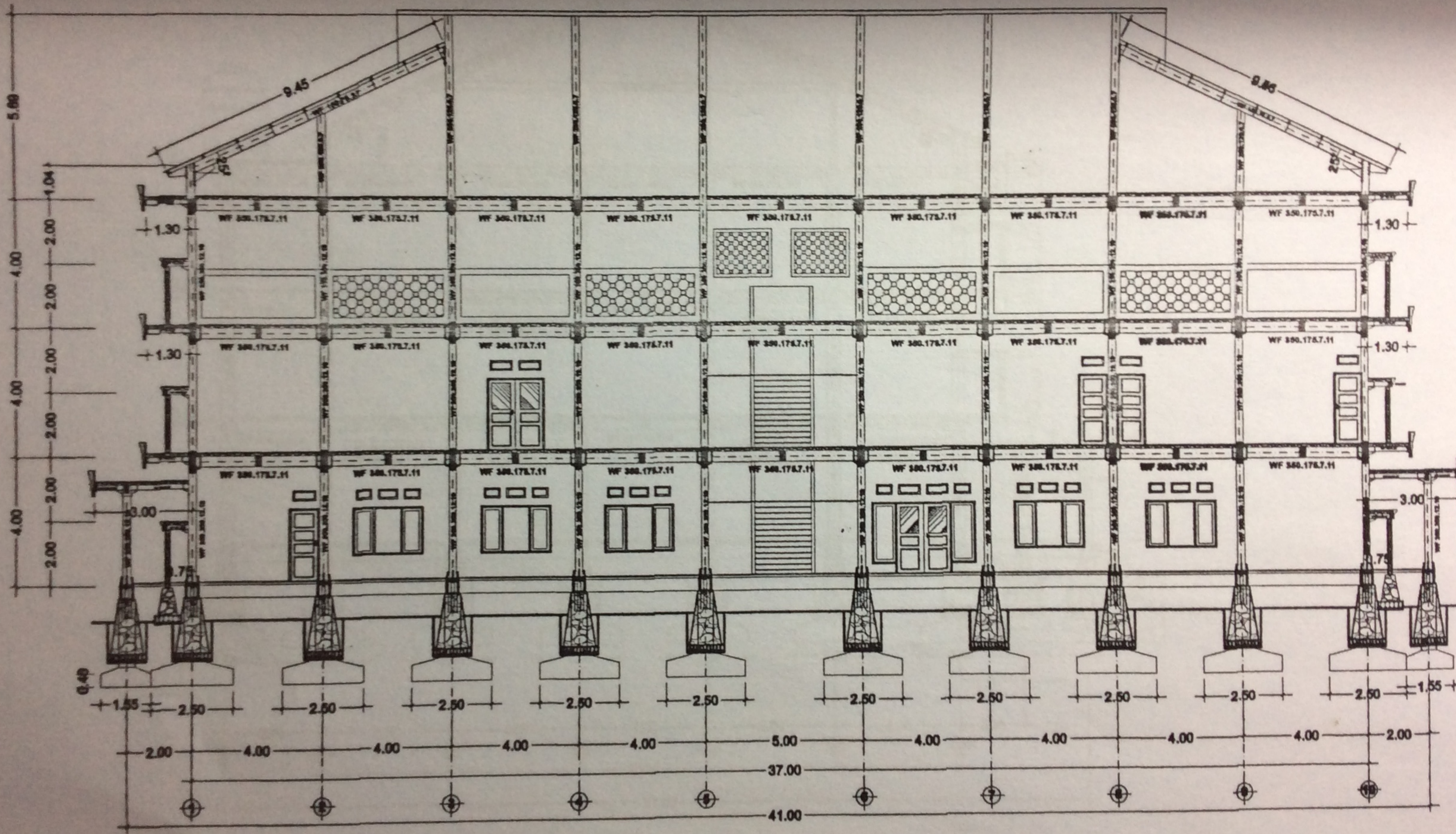
R POTONGAN A-A Skala 1 : 150
